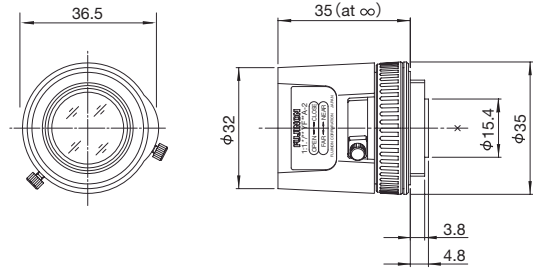
Unit : mm
